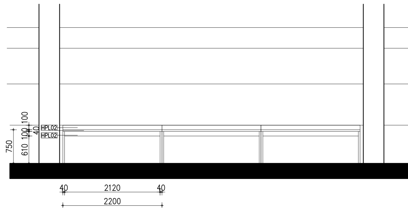
MW4 werktafels langs gevel verdieping 5 5x L=2200mm
